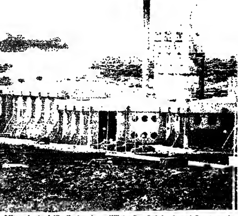
Mitten in der isländischen Lava-Wüste: Das Solekraftwerk Svartsengi
